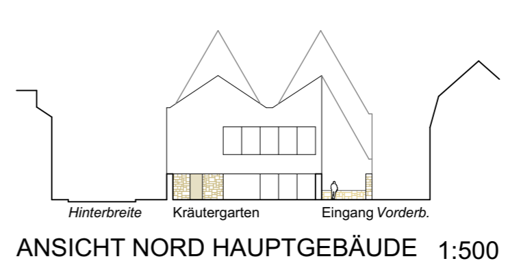
ANSICHT NORD HAUPTGEBÄUDE 1:500
