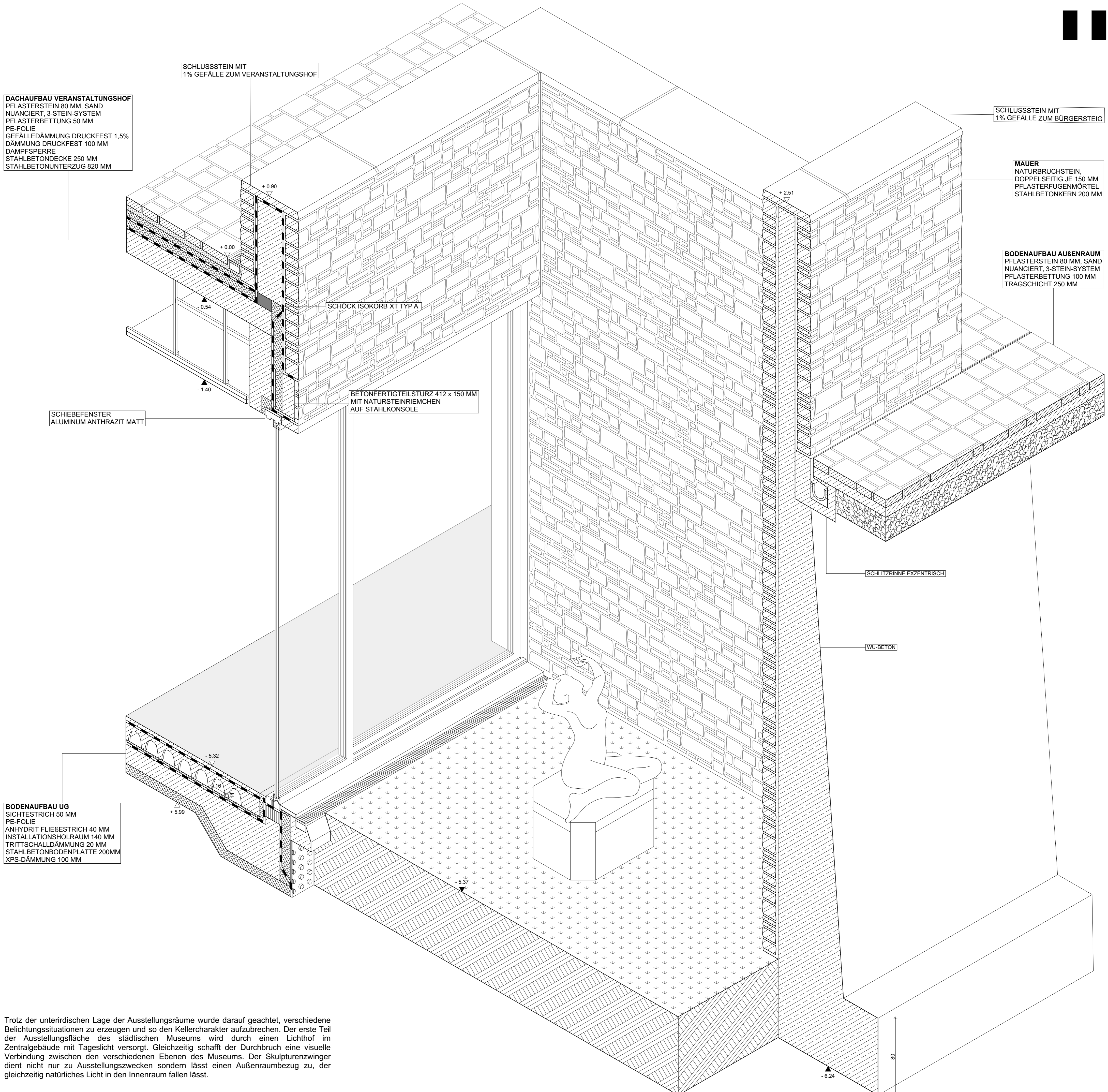
SNITTISOMETRIE LICHTGRABEN
