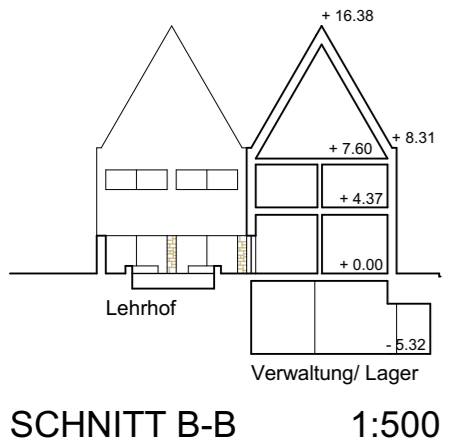
SCHNITT B-B 1:500
