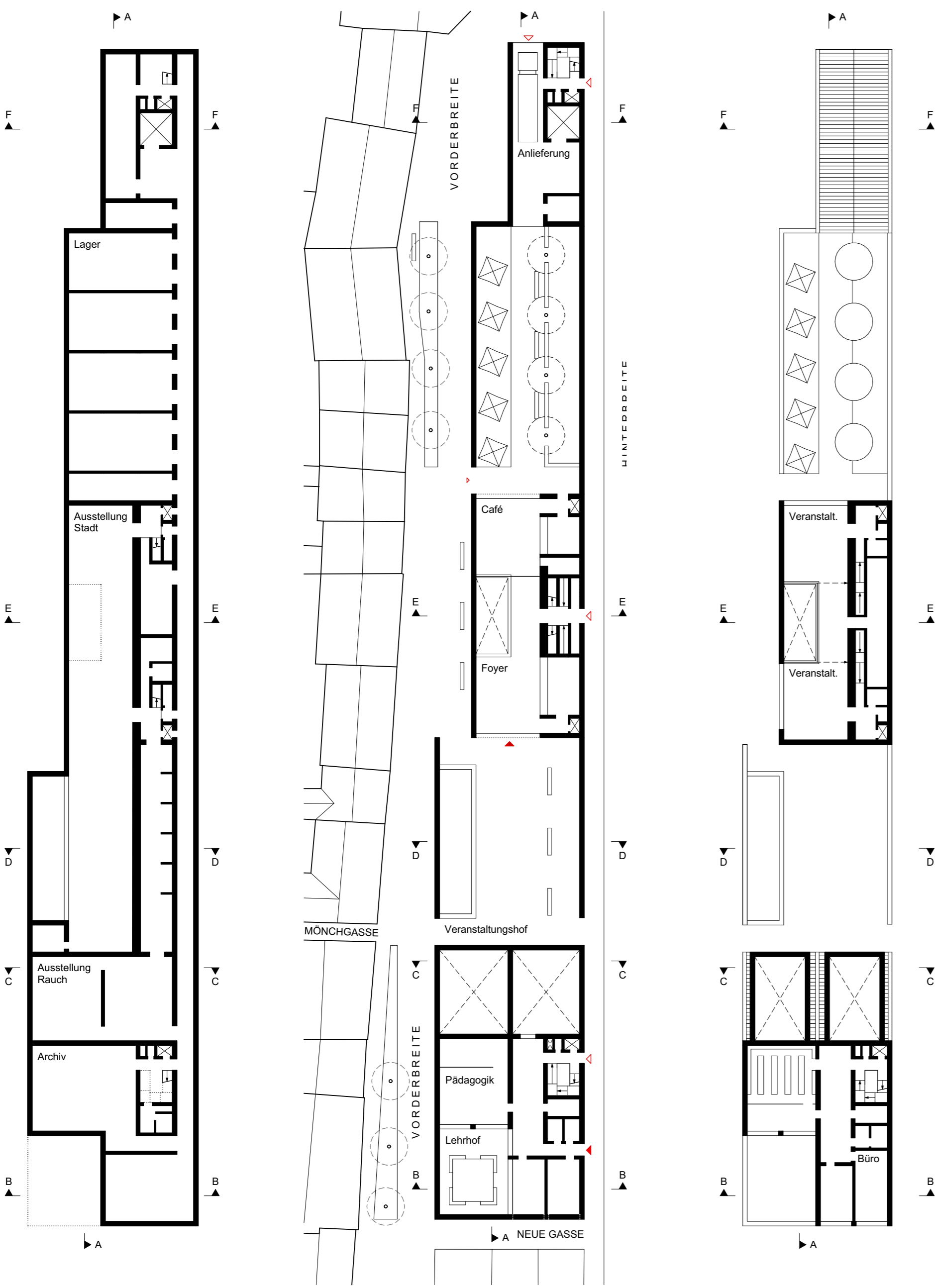
GRUNDRISS KG 1:500
