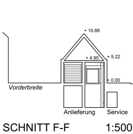
SCHNITT F-F 1:500
