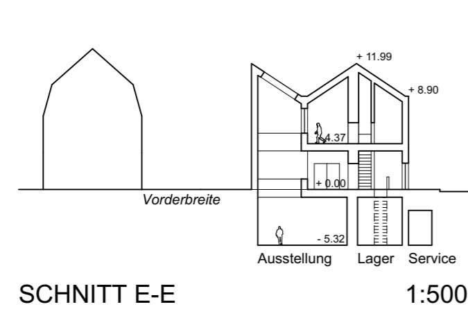
SCHNITT E-E 1:500
