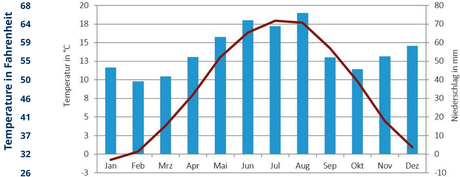
DWD Station Dresden-Klotzsche, Datenquelle DWD (228 müNN, 8,9 °C, 669 mm)
